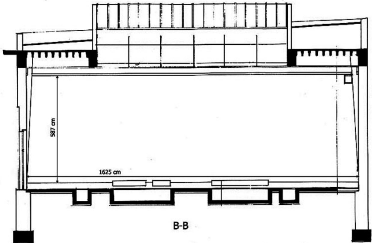
Paviljon - presek B-B
