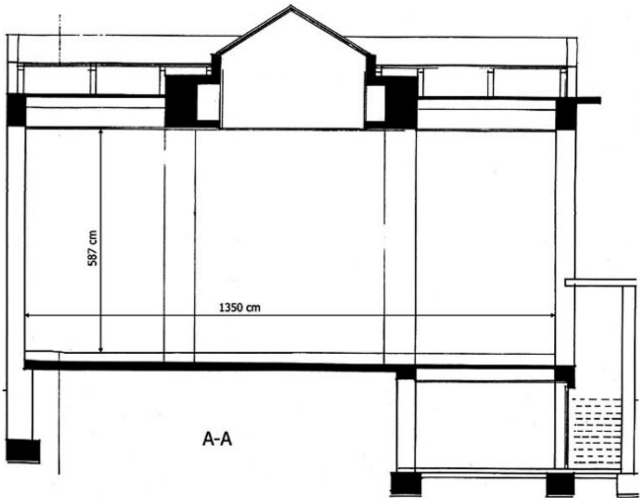
Paviljon - presek A-A
